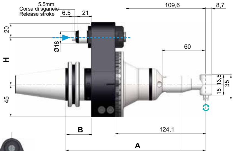
90° ANGLE SPINDLE RA - 200
